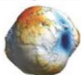
Физическая форма Земли
