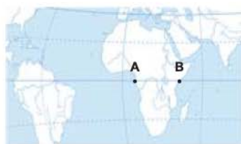
Разрывы, в результате заполнения которых возникают искажения.
