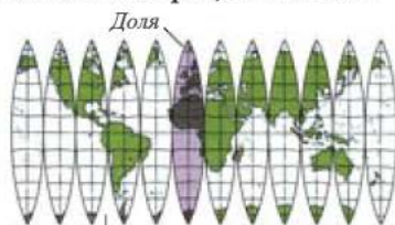
Разрывы, в результате заполнения которых возникают искажения.
