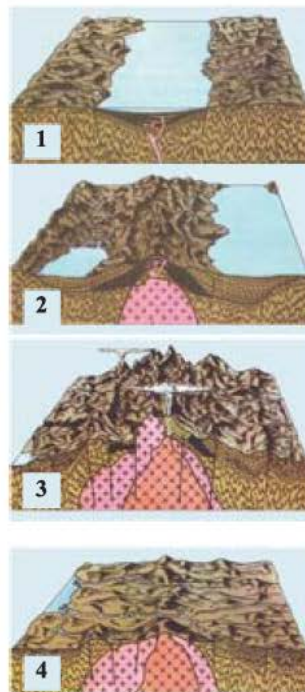
Этапы развития геосинклиналей
